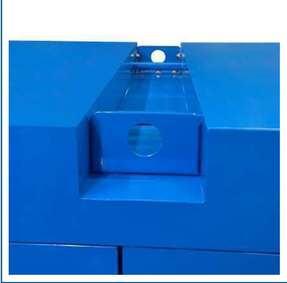
Cabina autoportante
